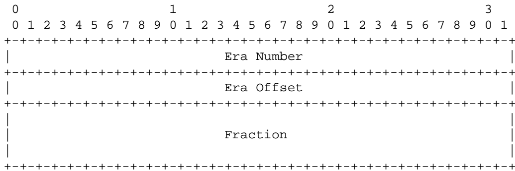
NTP Date Format
